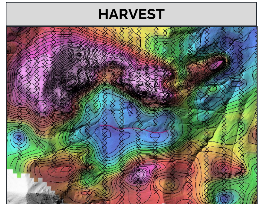
(Peak: 3.6 mGal)
