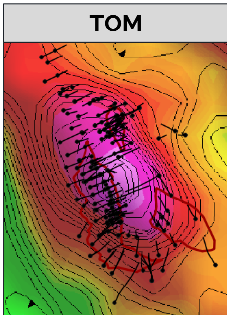
(Peak: 2.0 mGal)
