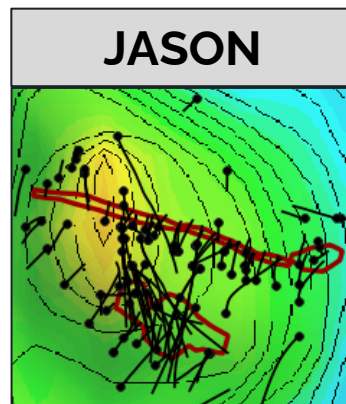
(Peak: 0.5 mGal)
